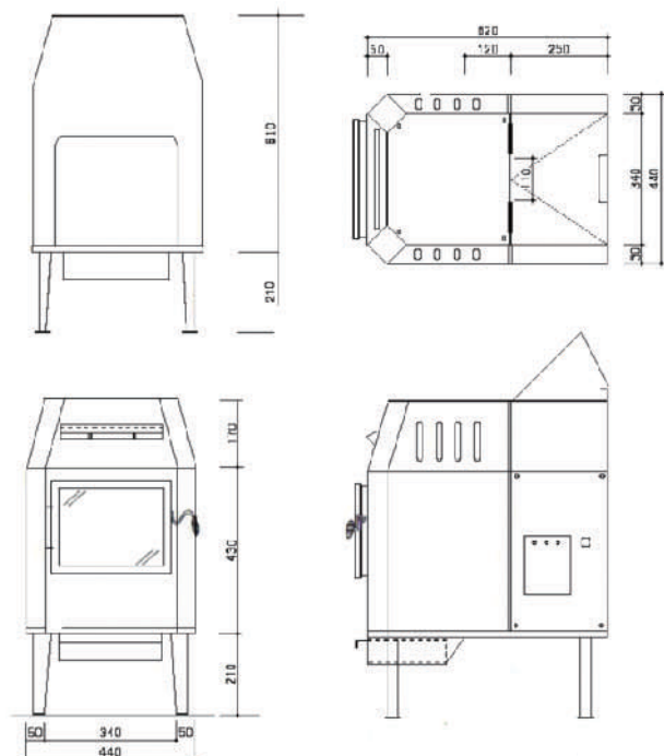
FF式 寸法図
